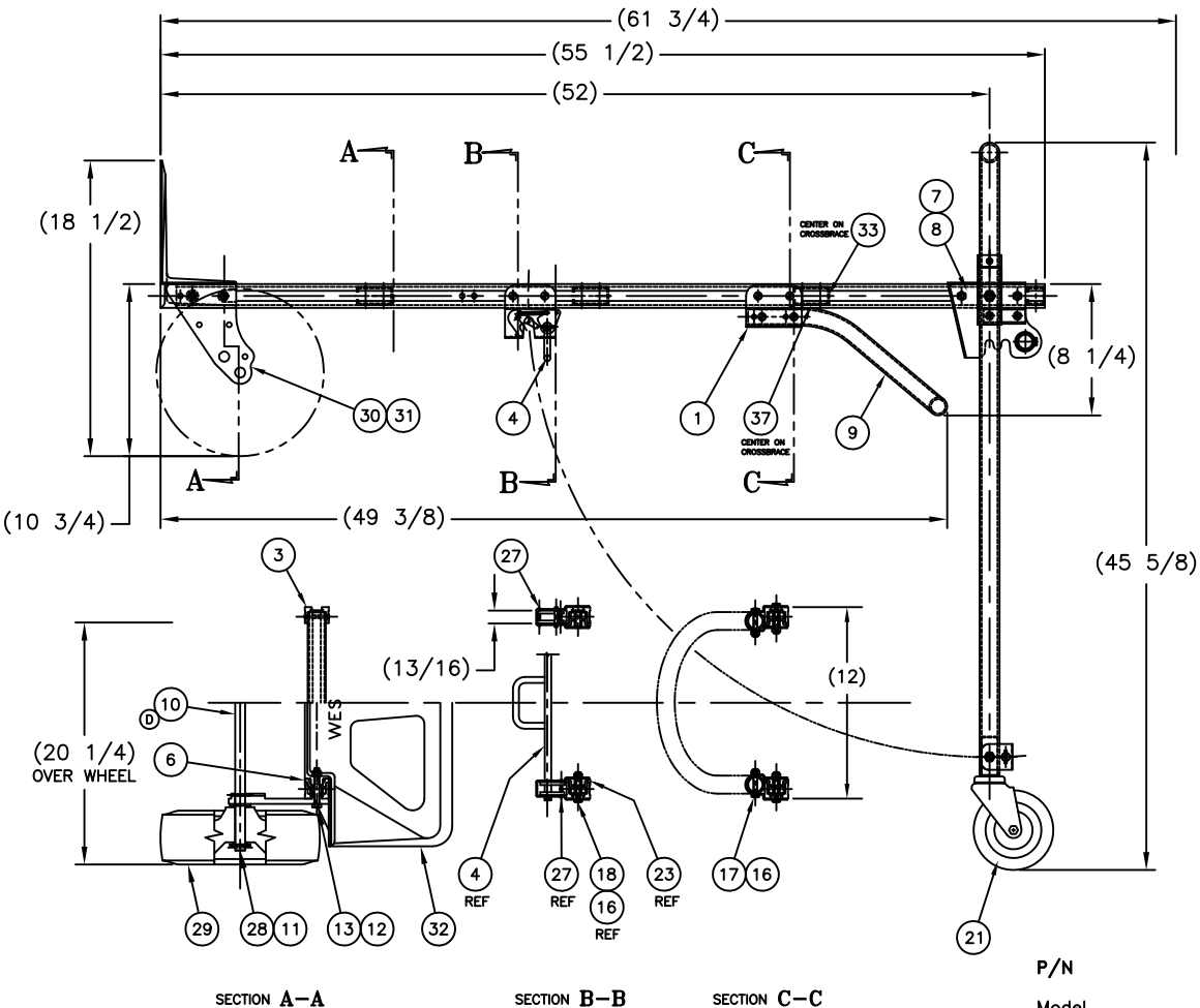
SECTION A-A
